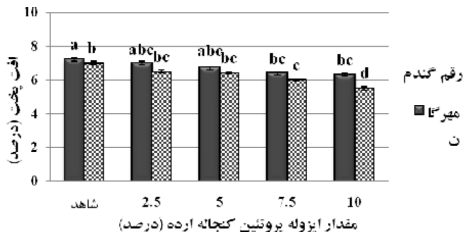
شکل 4- تأثیر افزودن ایزوله پروتئین کنجاله ارده به آرد حاصل از دو رقم گندم بهرنگ و مهرگان بر افت پخت (حروف مشابه از نظر آماری در P < 0.05 تفاوت معنی‌داری ندارند)
