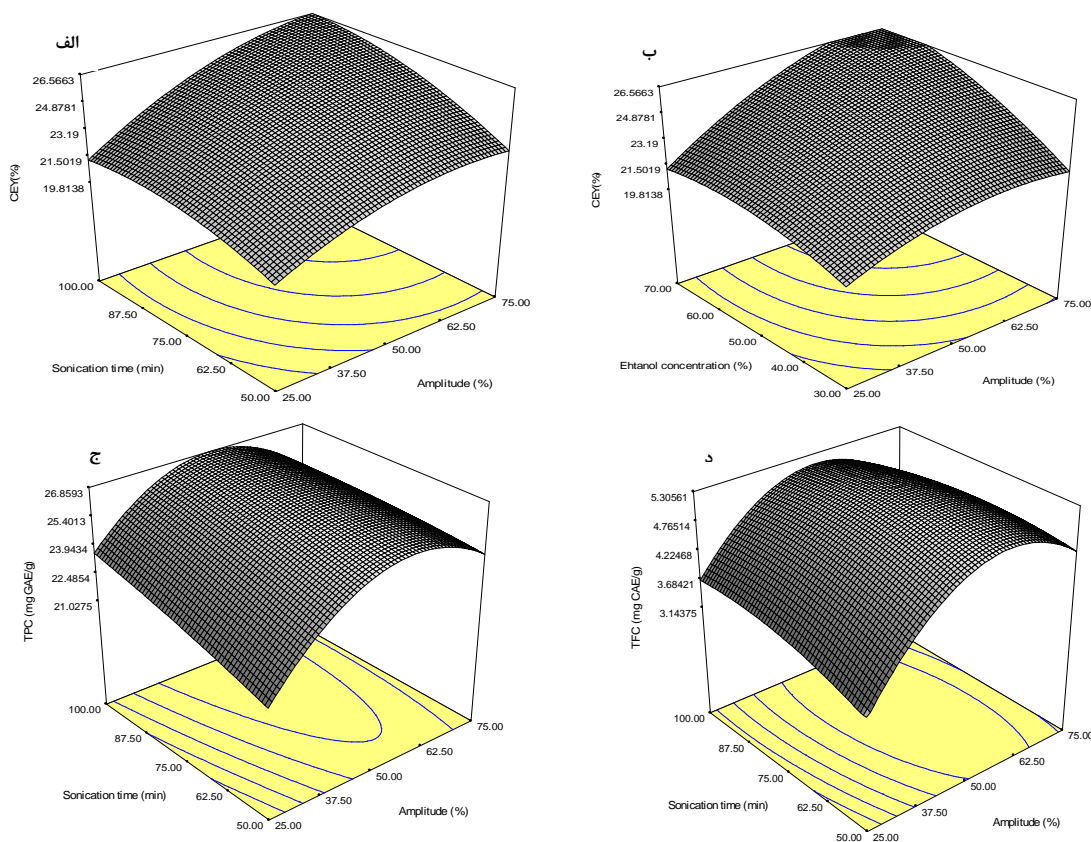
شکل 1- اثر شدت امواج فراصوت و مدت زمان اعمال فراصوت بر میزان استخراج عصاره خام (الف)، شدت امواج فراصوت و غلظت حلال اتانول بر میزان استخراج عصاره خام (ب)، شدت امواج فراصوت و مدت زمان اعمال فراصوت بر میزان ترکیبات کل فنولی (ج) و شدت امواج فراصوت و مدت زمان اعمال فراصوت بر میزان ترکیبات کل فلاونوئیدی (د).
