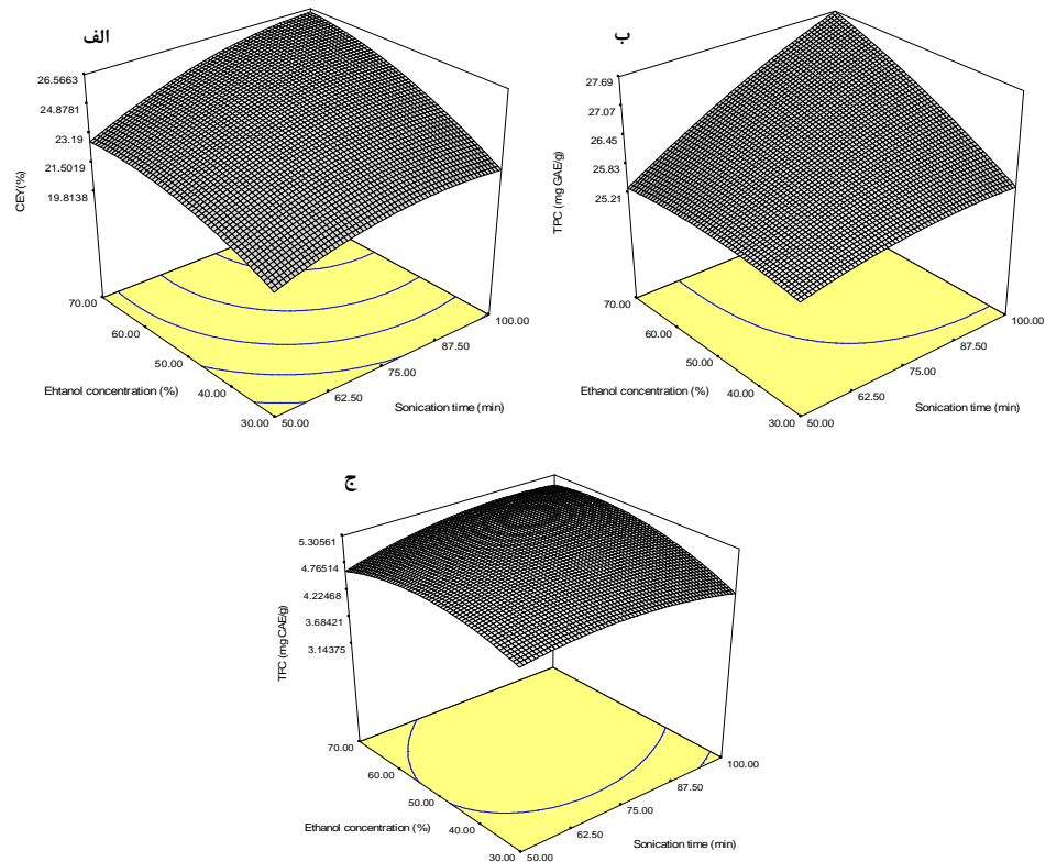
شکل 2- اثر مدت زمان اعمال فراصوت و غلظت حلال اتانول بر میزان استخراج عصاره خام (الف)، اثر مدت زمان اعمال فراصوت و غلظت حلال اتانول بر میزان ترکیبات کل فنولی (ب) و مدت زمان اعمال فراصوت و غلظت حلال اتانول بر میزان ترکیبات کل فلاونوئیدی (ج).
