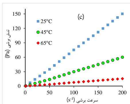
شکل 1: رئوگرام تنش برشی در مقابل سرعت برشی کنسانتره توت سفید در دما و غلظت‌های مختلف (a: 45 °Brix, b: 55 °Brix, and c: 65 °Brix)
