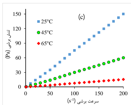
شکل 1- رئوگرام تنش برشی در مقابل سرعت برشی کنسانتره توت سفید در دما و غلظت‌های مختلف
