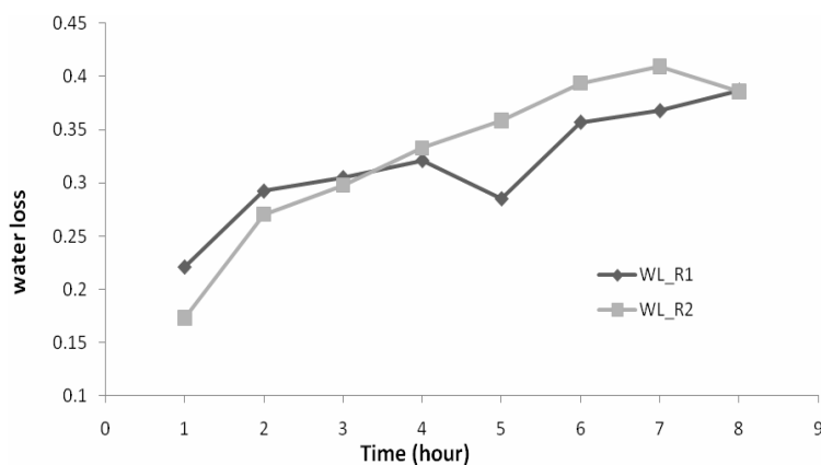
شکل ۲- تغییرات دفع آب (WL) در دو نسبت مواد جامد به مایع R_1=1:5 و R_2=1:10 (%w/w)
