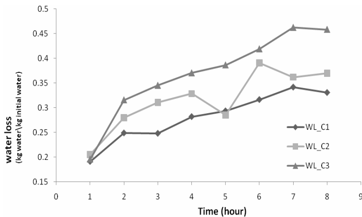
شکل ۳- تأثیر غلظت محلول اسمزی ساکارز ( C_1=50\% BX , C_2=60\% BX , C_3=70\% BX ) بر تغییرات دفع آب (WL)
