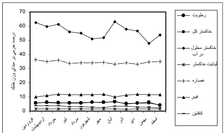
شکل ۲- روند تغییرات ویژگی‌های فیزیکوشیمیایی چای سیلان در
