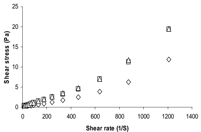
شکل ۳ - نمودار سرعت برشی - تنش برشی امولسیون‌ها در غلظت‌های مختلف پروتئین آب پنیر (۱۰٪، ۱۵٪، ۲۰٪، ۲۵٪) و زمان هموژنیزاسیون ۶ دقیقه.
