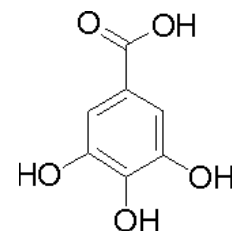
شکل ۱- ساختمان شیمیایی اسید گالیک (۱۴).
