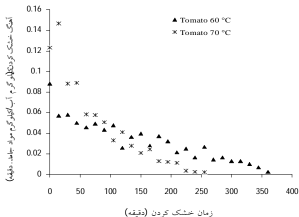
شکل 4- تغییرات آهنگ خشک کردن در مقابل زمان در دماهای مختلف در طی خشک کردن هوای داغ
