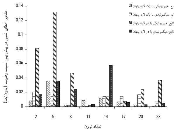
شکل 6- تغییرات مقادیر خطای نسبی در پیش‌بینی نسبت رطوبت با تغییرات نرون‌ها
