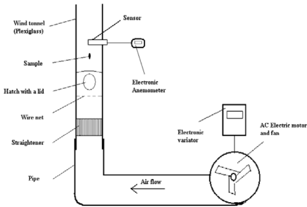
شکل ۱- دستگاه آزمایشگاهی مورد استفاده برای اندازه‌گیری سرعت حد نمونه‌های دانه‌ی جو
