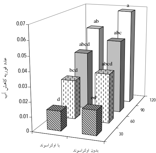
شکل 8 - اثر متقابل پیش تیمار اولتراسوند و زمان غوطه وری روی عدد فوریه کاهش آب
