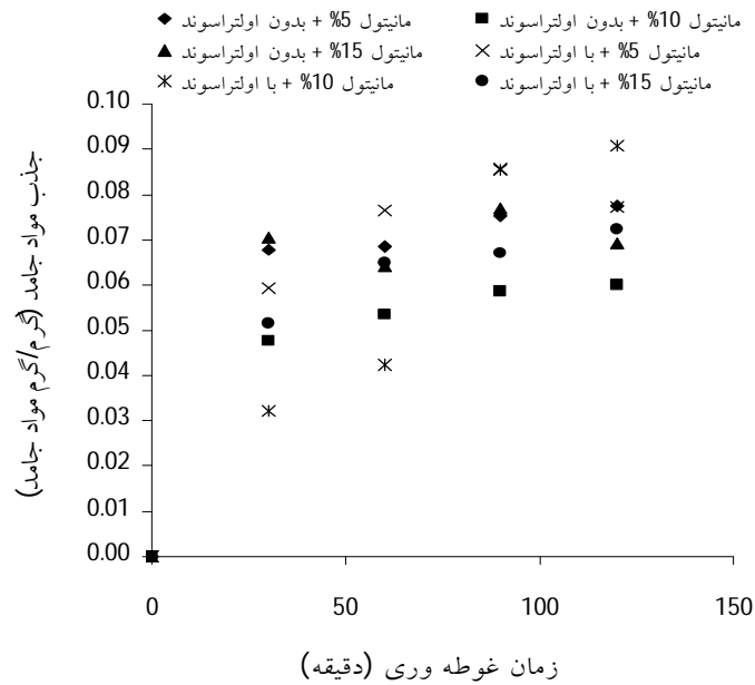
شکل 3- تاثیر پیش تیمار اولتراسوند بر روند تغییرات درصد جذب مواد جامد برش‌های ترب در طول زمان
