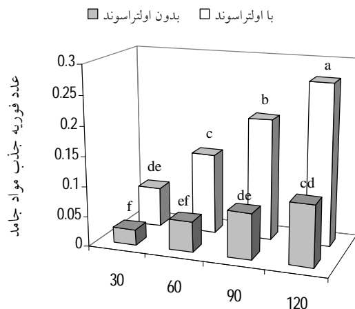
شکل 6 - اثر متقابل پیش تیمار اولتراسوند و زمان غوطه‌وری روی عدد فوریه‌ی جذب مواد جامد
